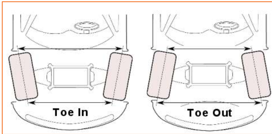
Fig 4.3.177: Toe-in/Toe-out
