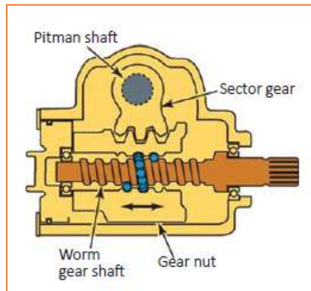
Fig 4.3.154: Steering gears
