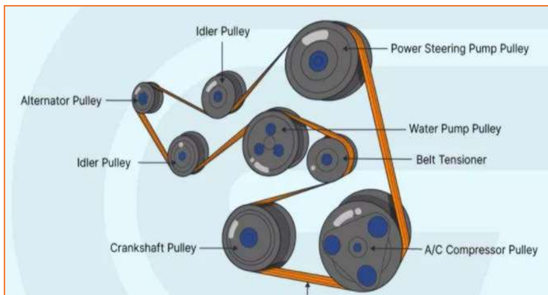
Fig 4.3.143: Fan belt layout
