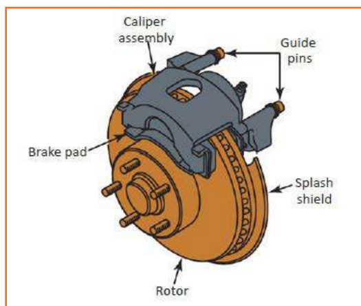
Fig 4.3.186: Disk brake
