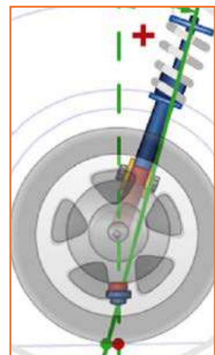
Fig 4.3.174: Castor Angle
