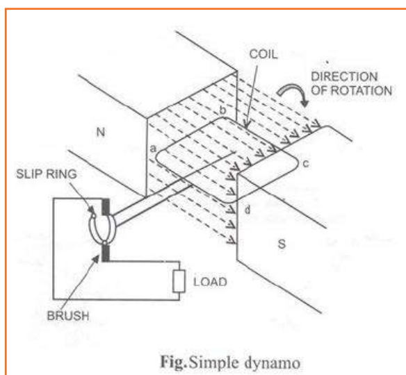
Fig 4.3.250: Simple dynamo
