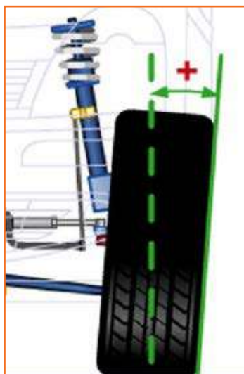
Fig 4.3.176: Camber Angle
