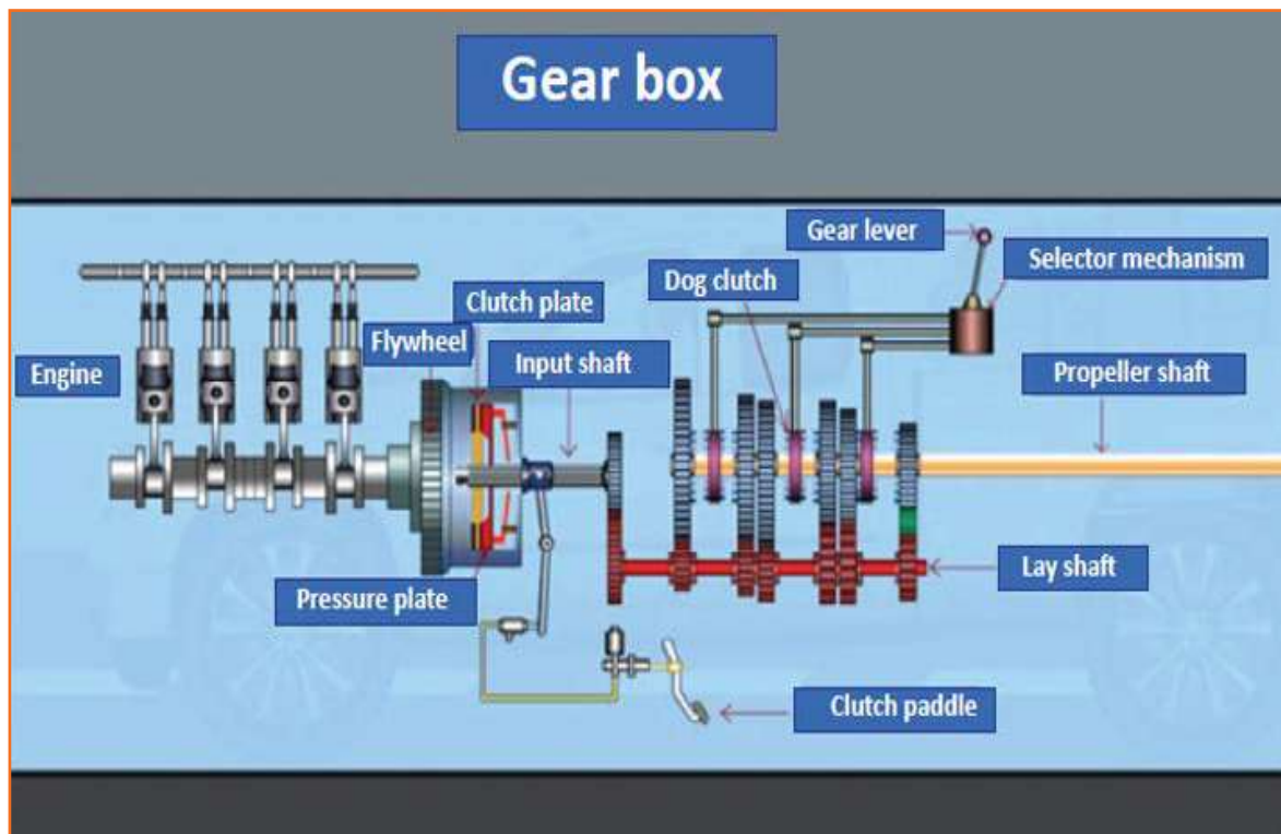
Fig 4.3.81: Gear box
