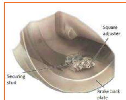
Fig 4.3.218: Wedge adjuster
