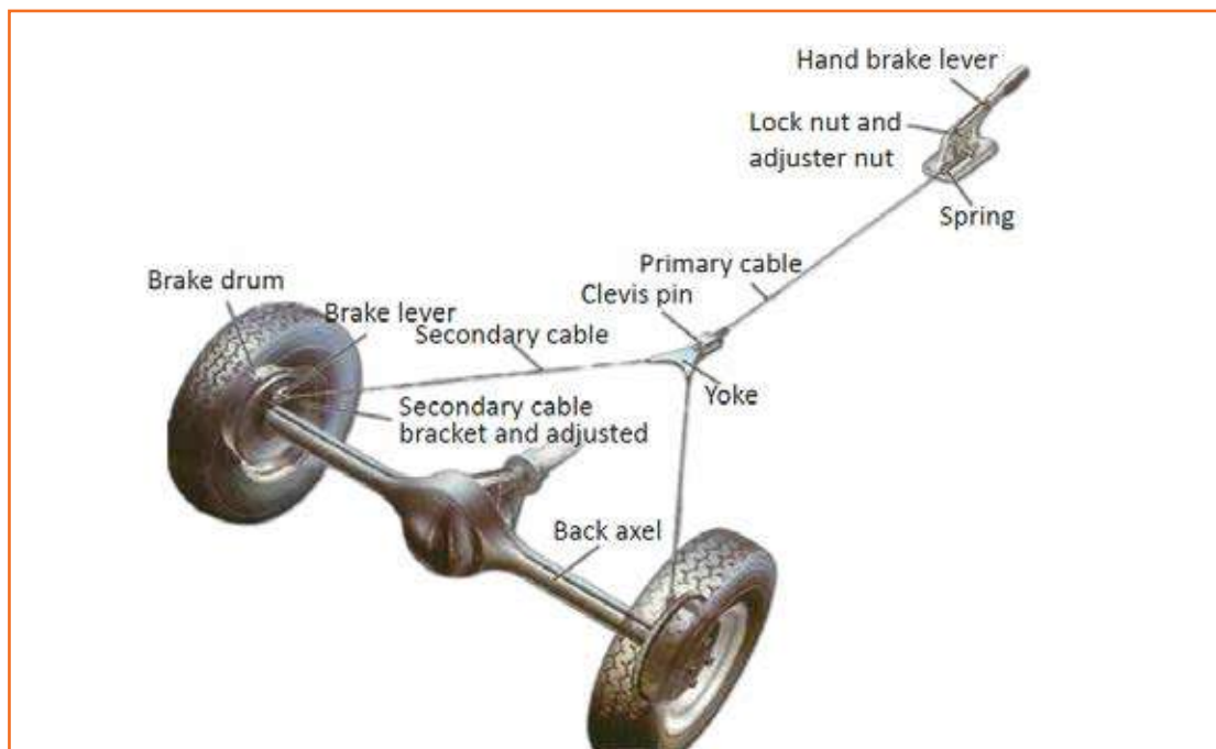
Fig 4.3.242: The handbrake
