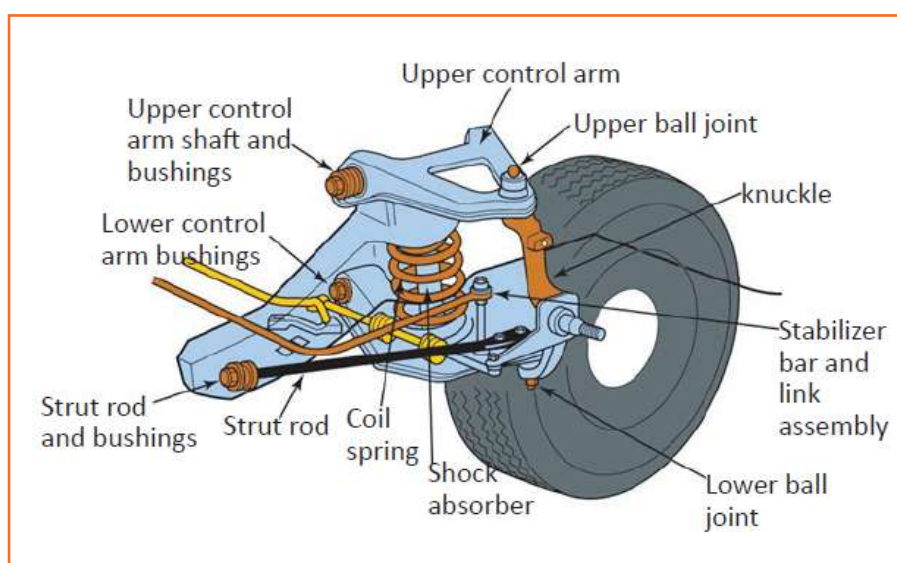
Fig 4.3.130: Strut rod
