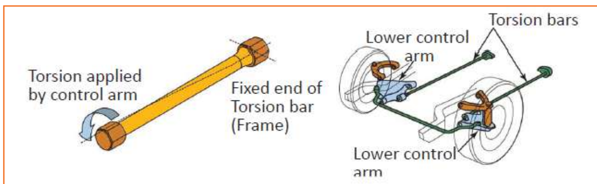
Fig 4.3.127: Torsion bar
