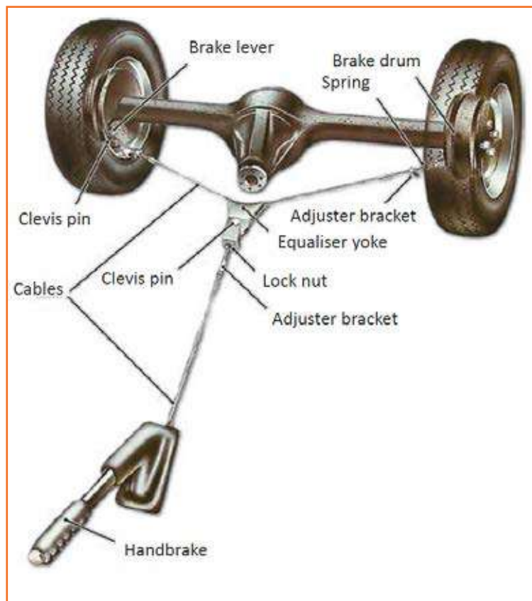
Fig 4.3.198: Handbreak layout
