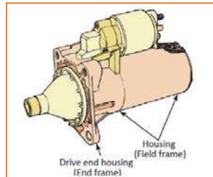
Fig 4.3.275: Motor
