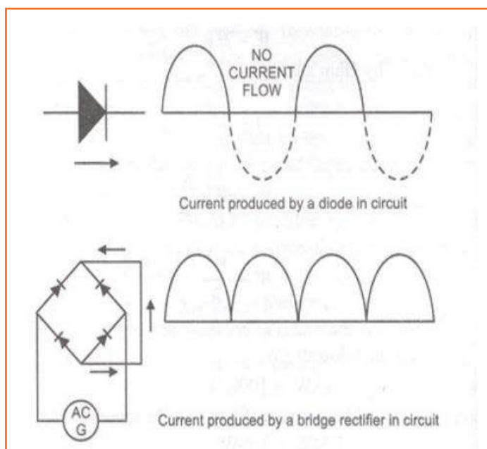
Fig 4.3.258: Rectifier
