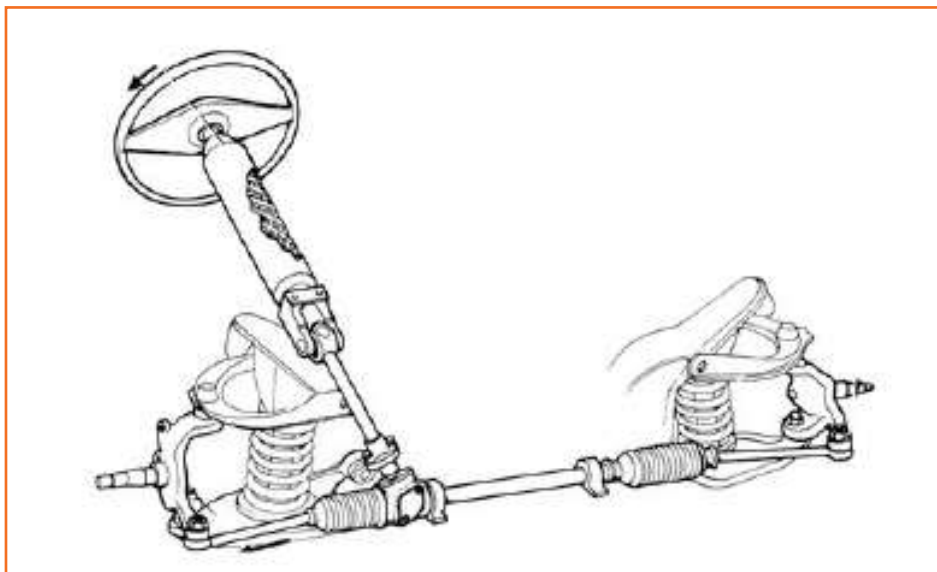
Fig 4.3.151: Steering linkages
